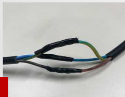
2. Isolar a emenda com fita isolante convencional
