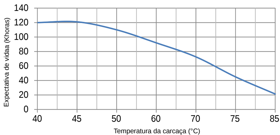
Expectativa de vida VS Temperatura da carcaça
