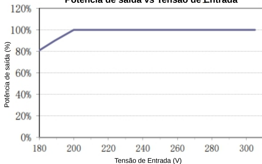
Potência de saída vs Tensão de Entrada
