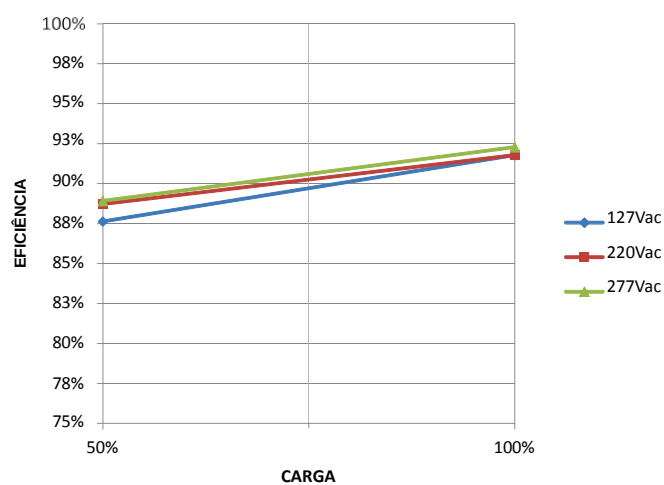
L4026-CIP4U1400/105P ( I_o=1,05A )
