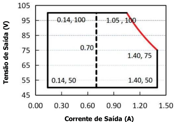
Tensão de Saída vs. Corrente de Saída
