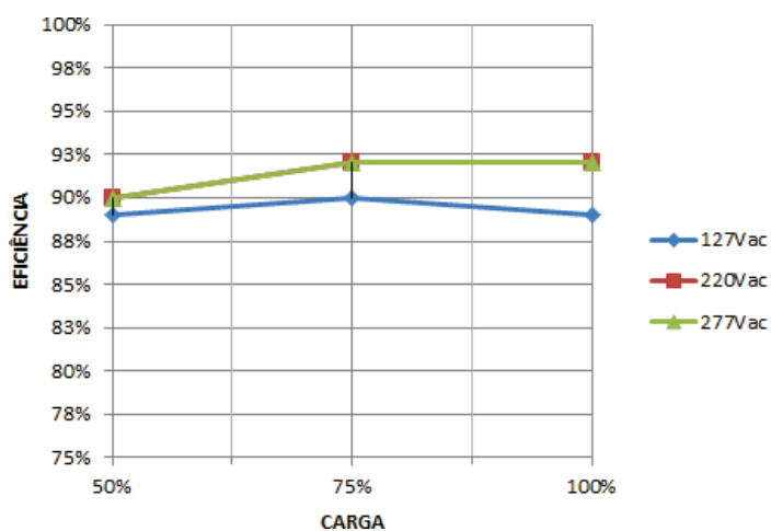
L4013-CIP4U1050/105P ( I_o=0,7A )
