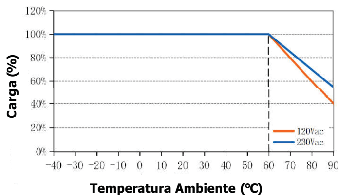
Carga vs. Temperatura Ambiente
