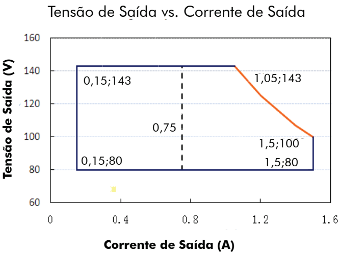
L4015-CIP4U1500/150P
