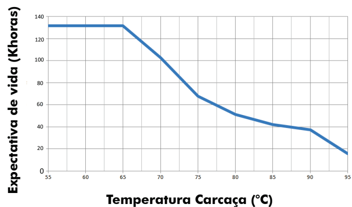
Expectativa de Vida vs. Temperatura Carcaça (Tc)
