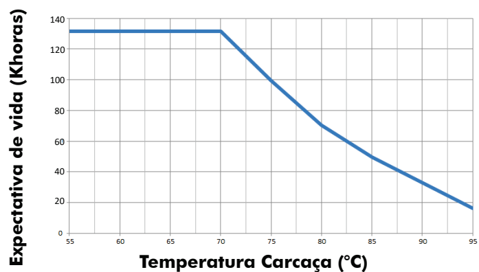
Expectativa de Vida vs. Temperatura Carcaça (Tc)
