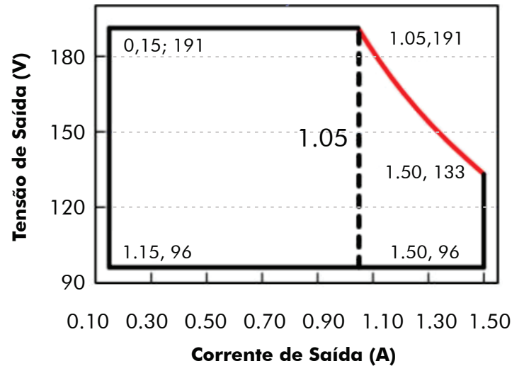
Tensão de Saída vs. Corrente de Saída
