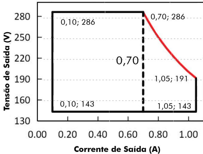
Tensão de Saída vs. Corrente de Saída
