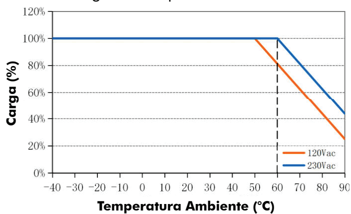
Carga vs. Temperatura Ambiente
