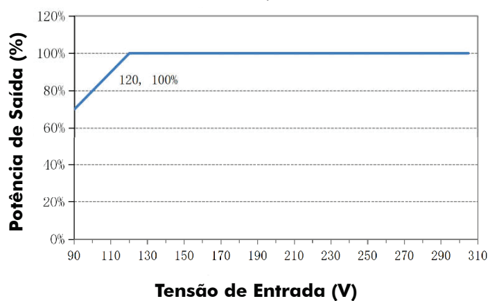
Potência de Saída vs. Tensão de Entrada
